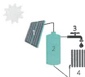
1. Zonnecollector | 2. Opslagvat zonneboiler | 3. Sanitair warm water | 4. Afgifta-element voor ruimteverwarming (radiator)
